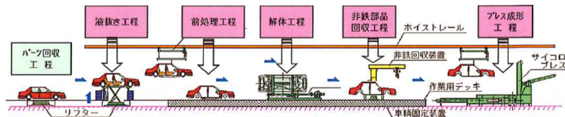
図2. 西日本オートリサイクル(株)の精緻解体プロセス
