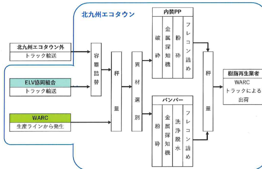
図3. 北九州エコタウン企業連携による廃車由来樹脂リサイクルスキーム
